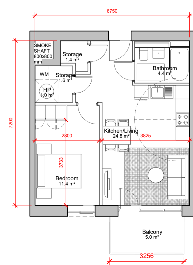
1 BED TYPE B5 1 : 100
