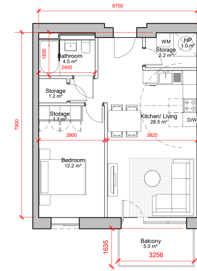
1 BED TYPE A3 1 : 100
