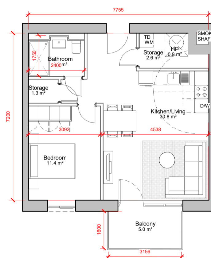
1 BED TYPE B2 1 : 100
