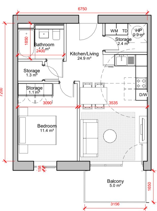
1 BED TYPE B 1 : 100
