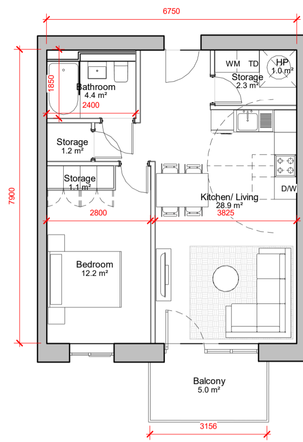
1 BED TYPE A 1 : 100
