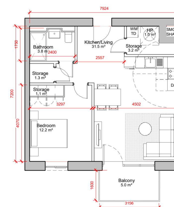
1 BED TYPE B3 1 : 100
