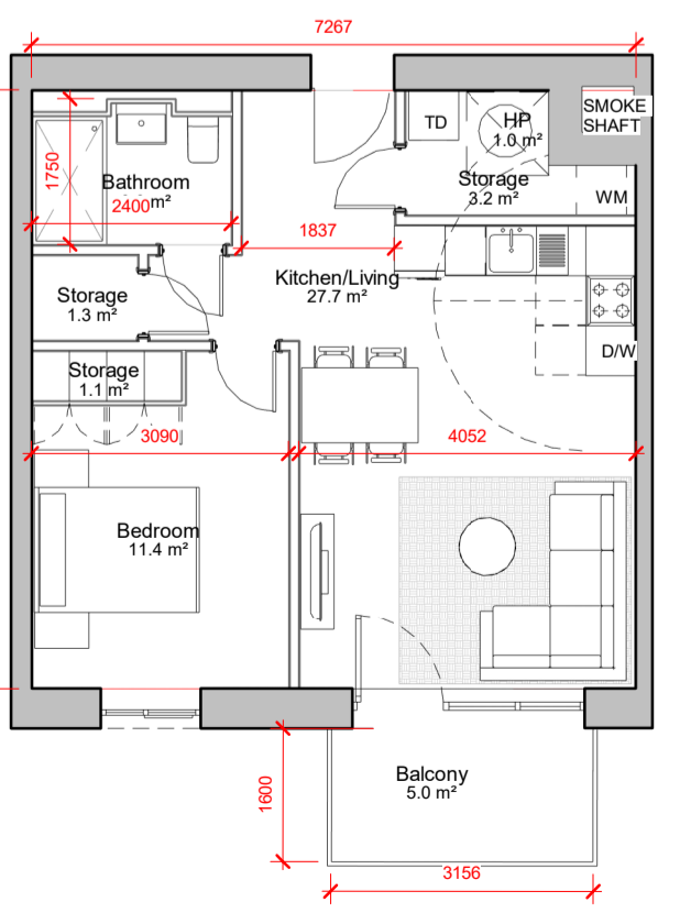
1 BED TYPE B4 1 : 100
