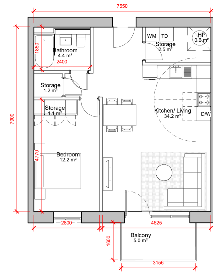
1 BED TYPE A2 1 : 100
